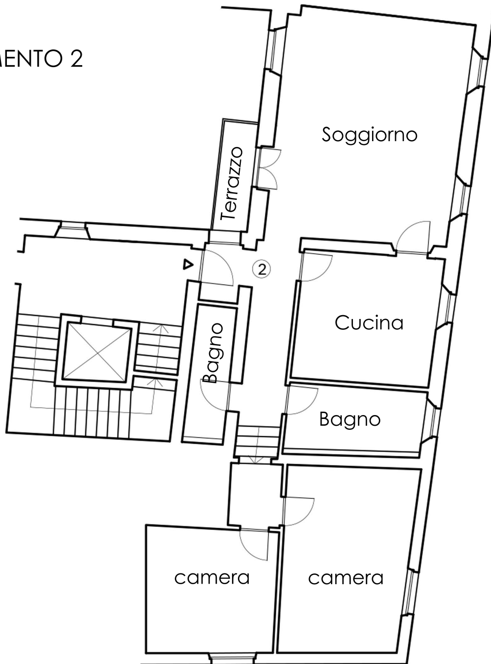
Piano primo
